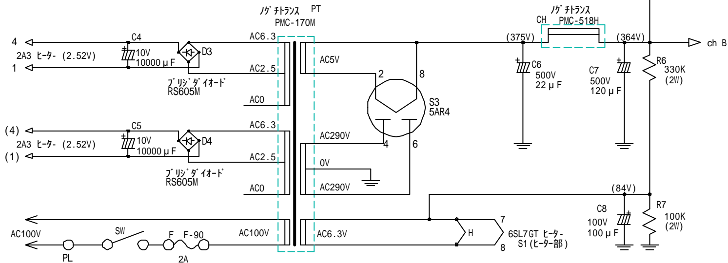
L (R) 2回路
